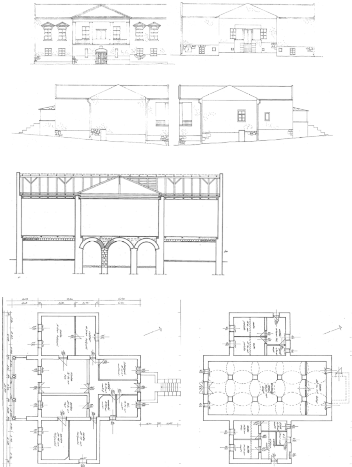
Waldbott-borház felmérése
