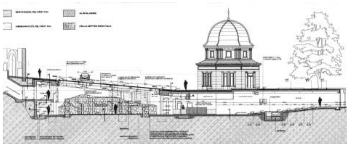
70. kép. A Cella Septichora Látogatóközpont engedélyezési tervének metszete a bejárat szintén keresztül.
