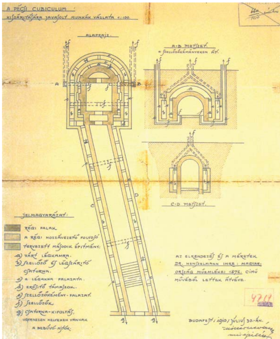
68. kép. Az 1. sz. (Péter-Pál) ókeresztény sírkamra Möller-féle védelmének terve, 1910.
